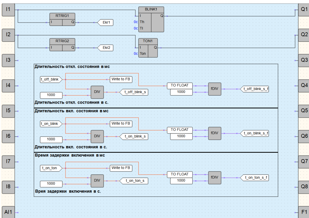
Рисунок 11.13 – Схема алгоритма
