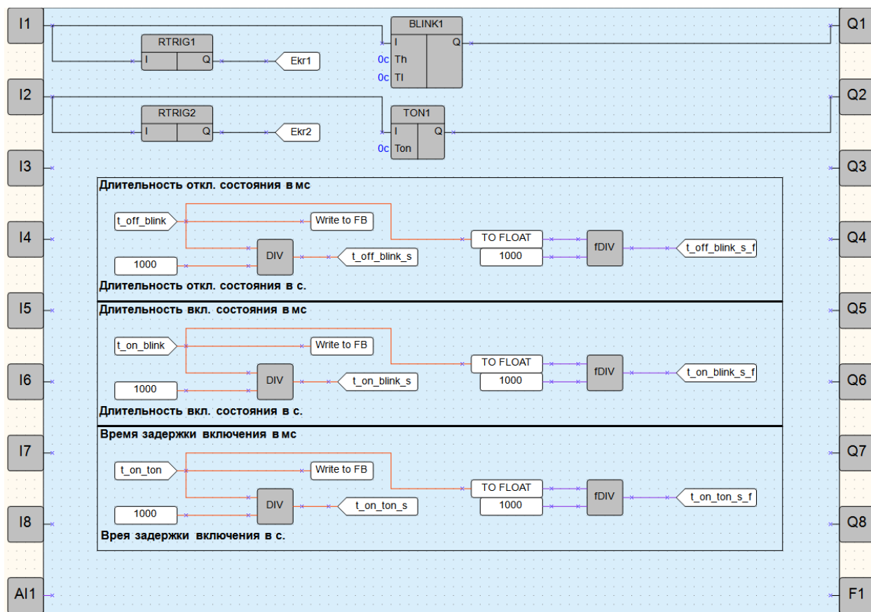
Рисунок 11.13 – Схема алгоритма
