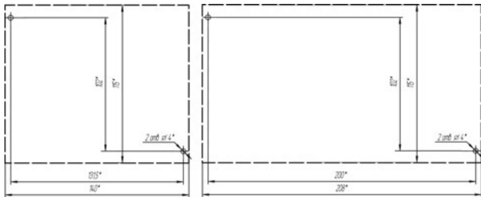
а) ПЛК110.X.30(32).X-X
