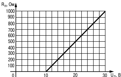
Рисунок 3.7 – График зависимости R_n от U_{п}
