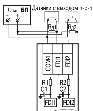
Рисунок 6.3 – Подключение к входам типа «ДС» датчиков с выходом n-p-n
