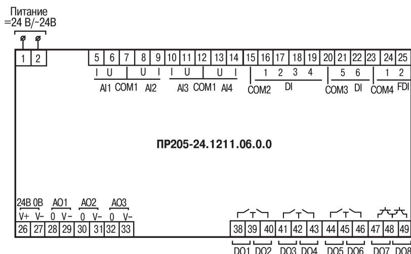
Рисунок А.7 – Расположение контактов для ПР205-24.1211.06.0.0
