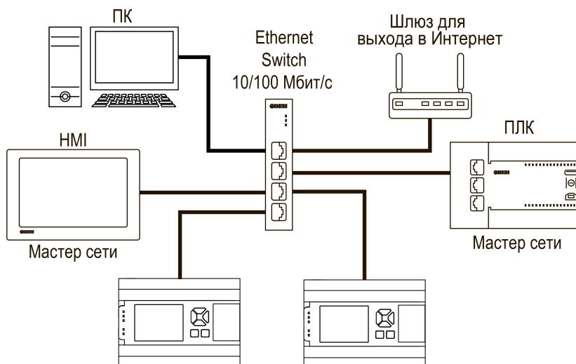
Рисунок 6.20 – Подключение по схеме «Звезда»
