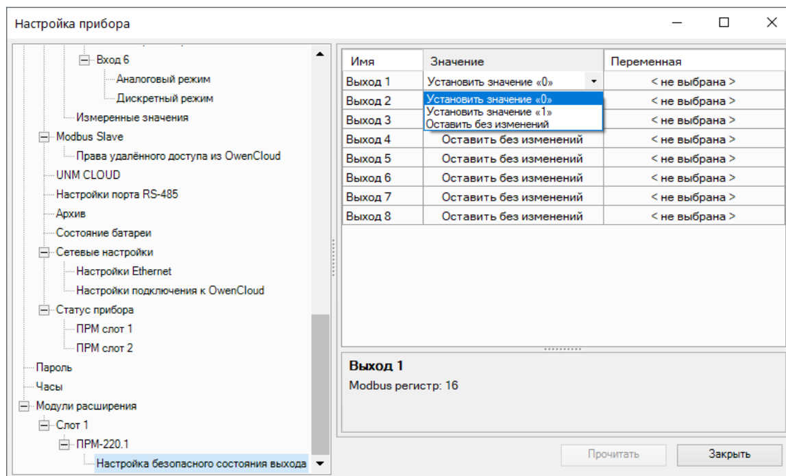
Рисунок 4.14 – Настройка безопасного состояния дискретных выходов ПРМ
