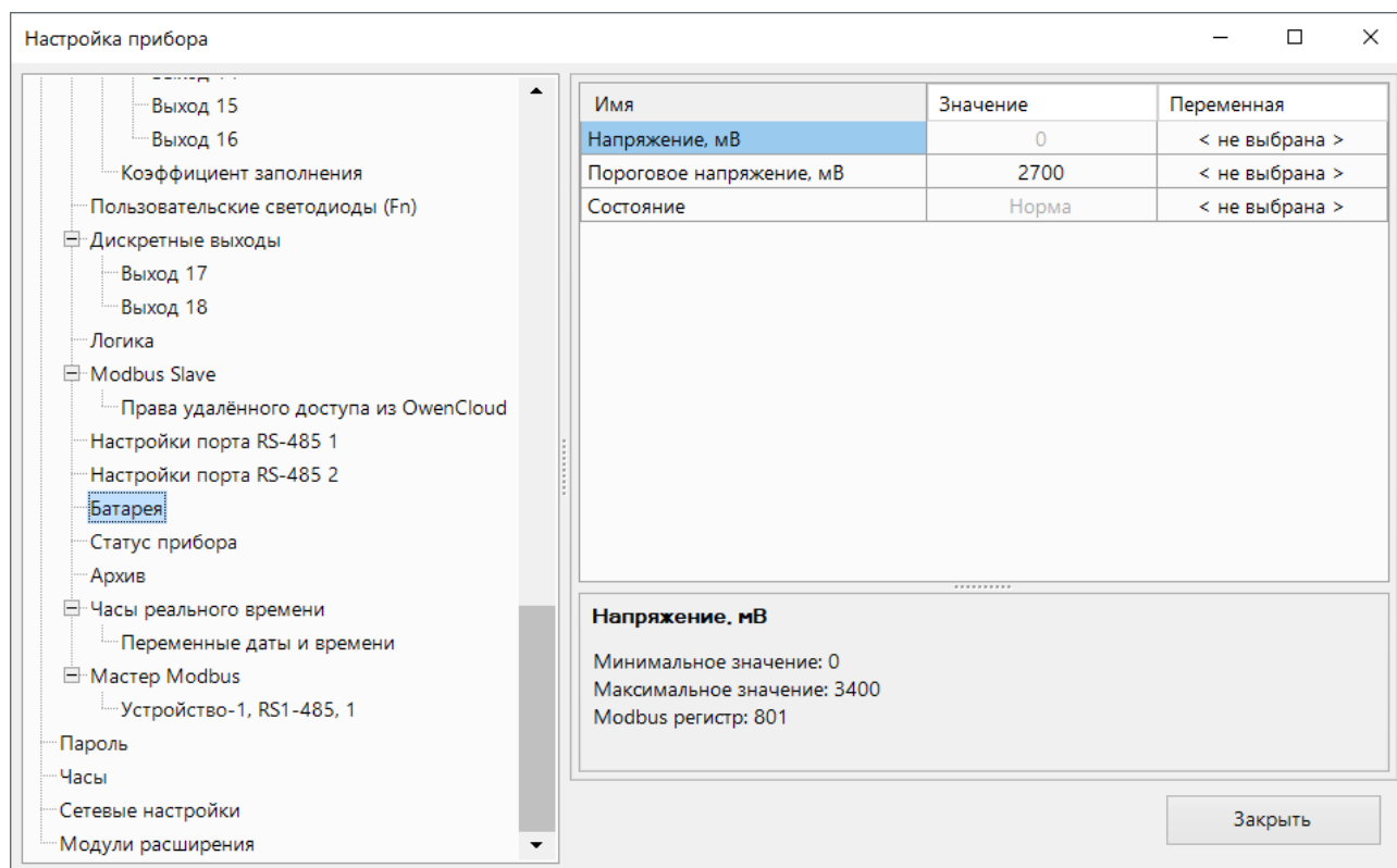
Рисунок 4.33 – Параметры состояния батареи
