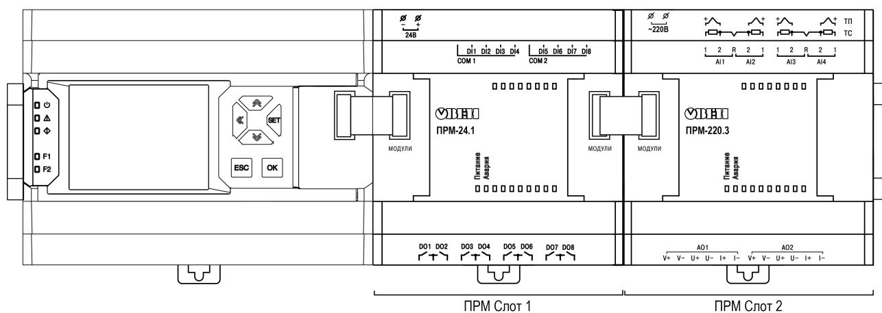
Рисунок 6.17 – Расположение модулей расширения на шине
