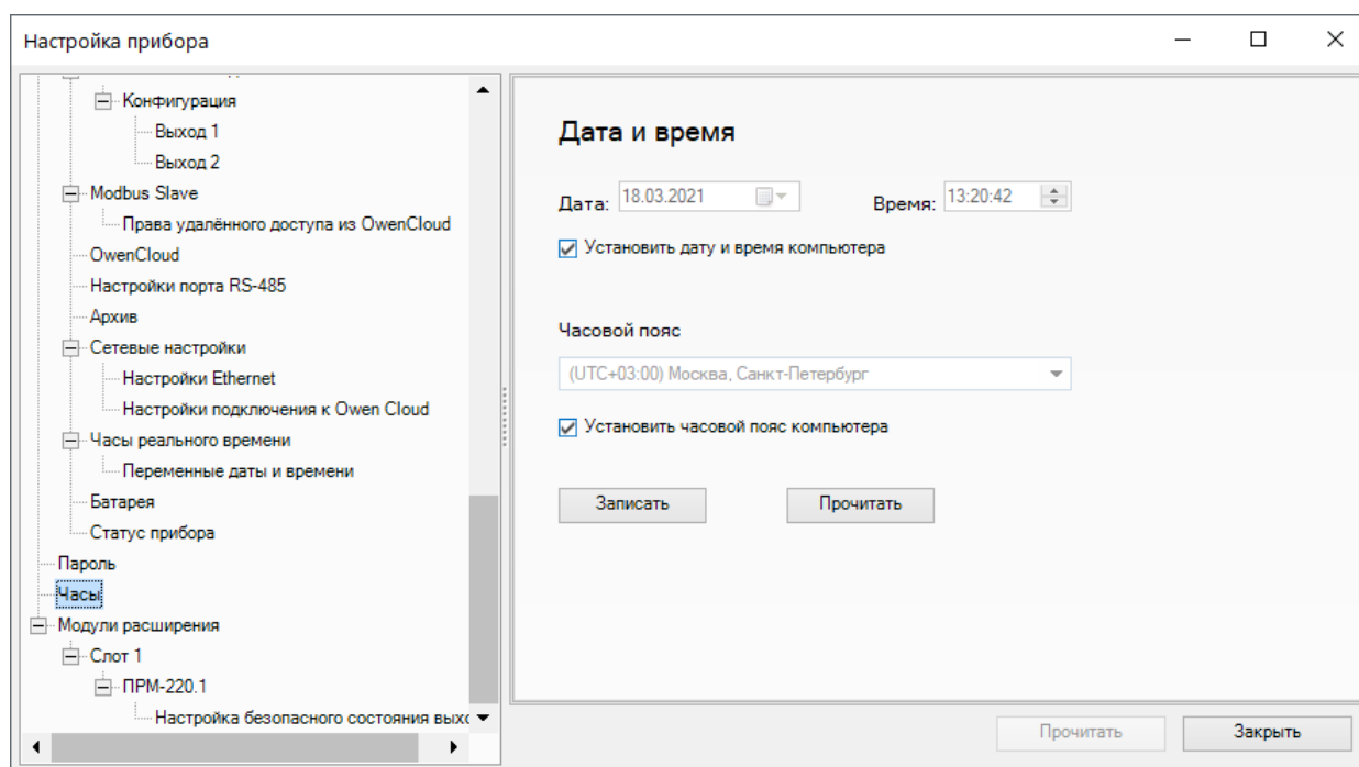
Рисунок 4.27 – Настройка значений даты и времени
