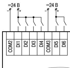
Рисунок 6.5 – Подключение к дискретным входам датчиков типа «сухой контакт» для сигналов постоянного тока =24 В
