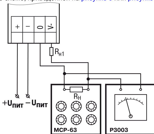
Рисунок В.3 – Схема подключения к ВЭ для юстировки сигналов типа «4...20 мА» ( R_H < 300
