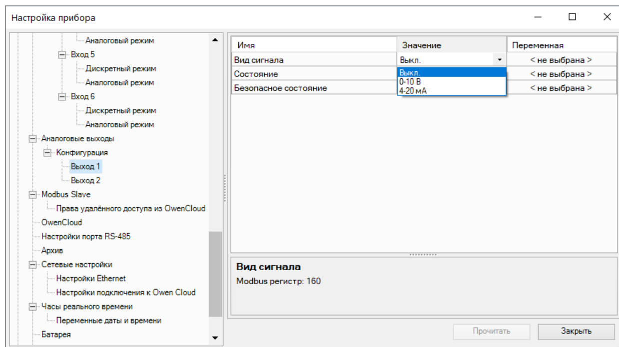
Рисунок 4.15 – Настройка универсальных аналоговых выходов
