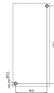
Рисунок 3 – Установочные размеры для монтажа на стену
