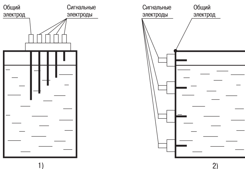
Рисунок 5.2 – Применение кондуктометрических зондов
