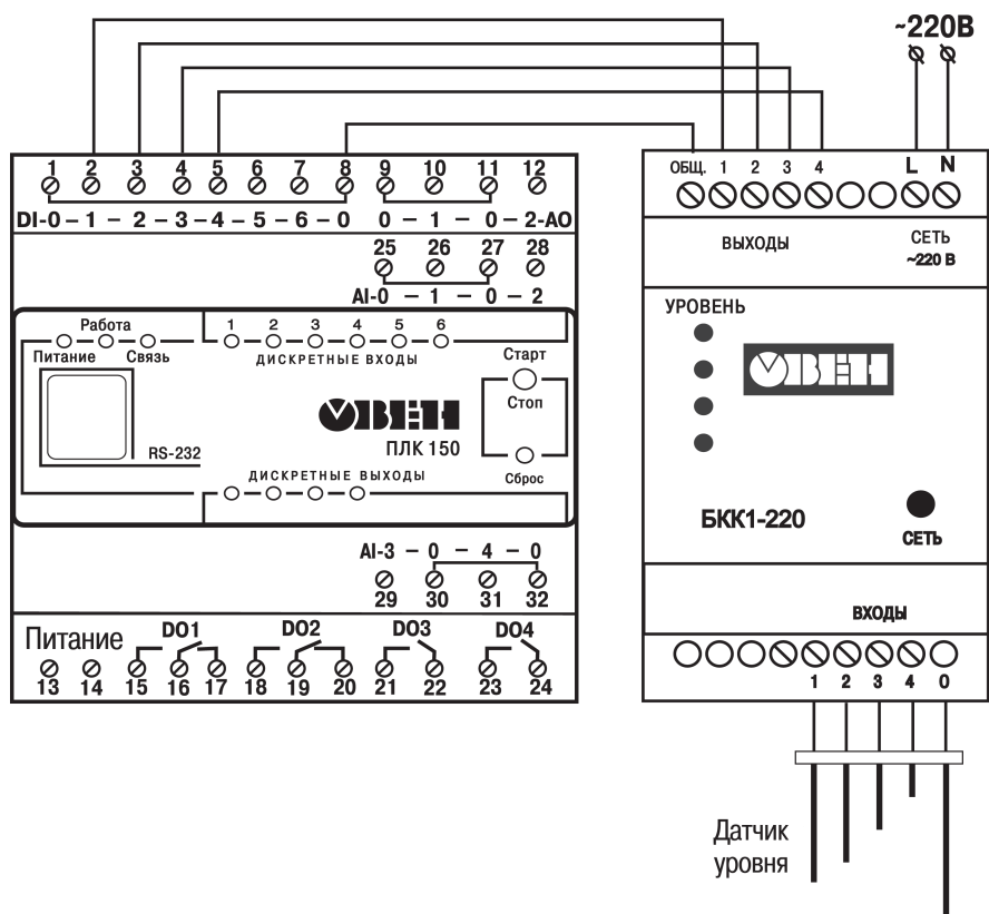
Рисунок 5.5 – Схема подключения БКК1-220 к ПЛК150-220
