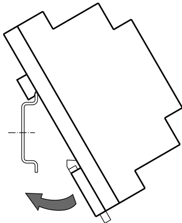
Рисунок 4.1 – Монтаж прибора на DIN-рейку
