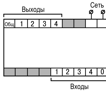
Рисунок 5.1 – Назначение клеммников
