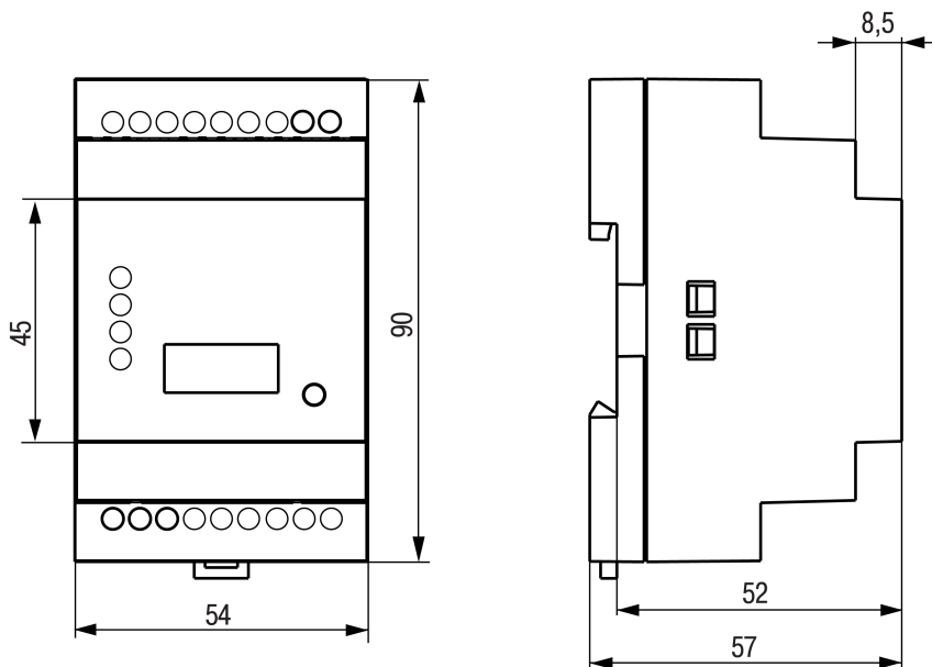
Рисунок 4.2 – Габаритные размеры прибора
