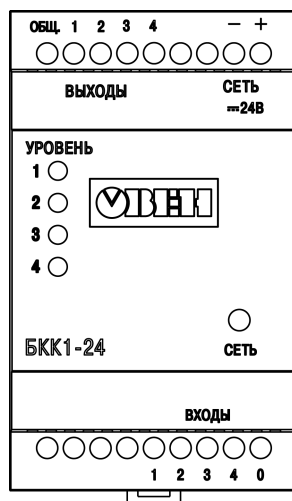
Рисунок 6.2 – Лицевая панель БКК1-24
