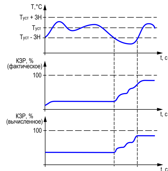
Рисунок 14.1 – Принцип работы КЗР
