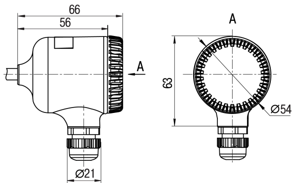
Рисунок В.1 – Габаритные размеры пластмассовой коммутационной головки
