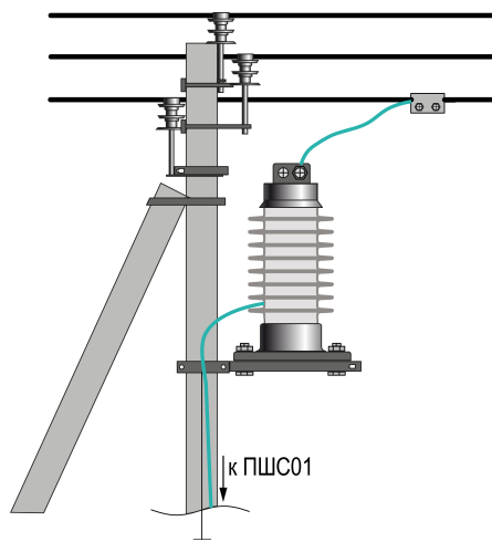
Рисунок 5.4 – Расположение УП-ПШС-10.О на опорах
