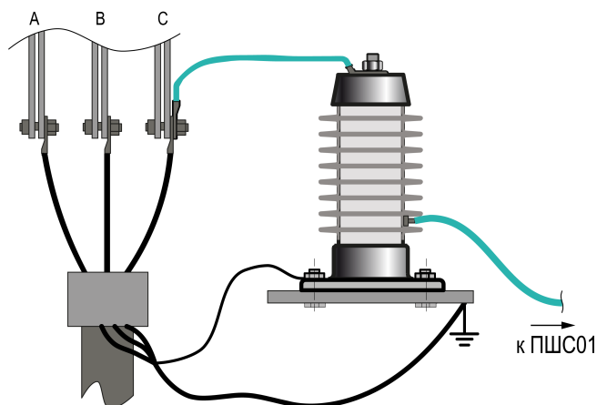
Рисунок 5.6 – Схема подключения УП-ПШС-10.0 в ячейке ввода напряжения 10 кВ
