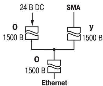
Рисунок 5.1 – Схема гальванической развязки
