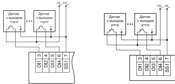
Рисунок 3 – Подключение датчиков с выходным транзистором п-р-п типа с открытым коллектором
