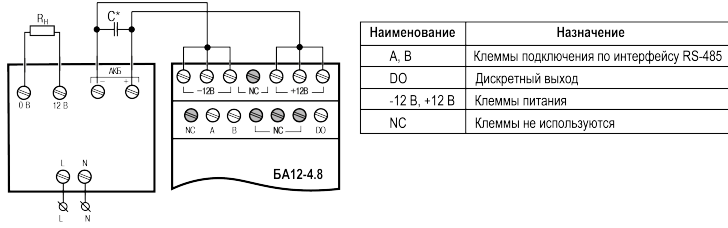
Рисунок 5.1 – Схема подключения
