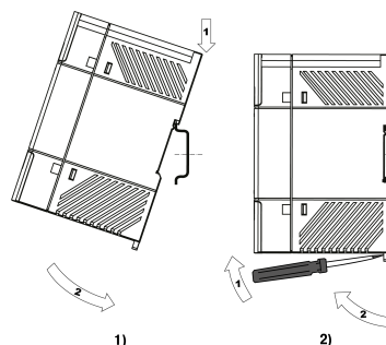
Рисунок 4.3 – Монтаж (1) и демонтаж (2) прибора
