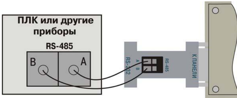
Рис. 6.1. Схема подключения интерфейса RSC485 для конфигурирования панели ИП320
