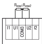
Рисунок 6 – Подключение резистивных датчиков
