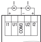
Рисунок 7 – Подключение датчиков с выходом в виде тока
