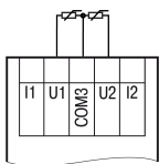
Рисунок 5 – Подключение ТС к AI
