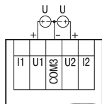
Рисунок 8 – Подключение датчиков с выходом в виде напряжения
