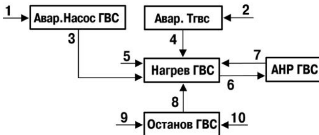
Рисунок 4.1 – Схема перехода между режимами контура ГВС
