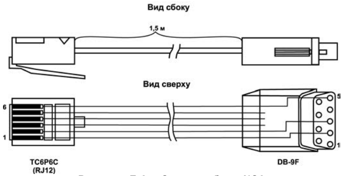
Рисунок Д.2 – Схема кабеля KC2
