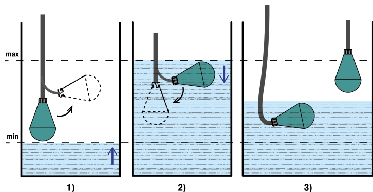
1) 2) 3) Рисунок 4.2 – Принцип действия
