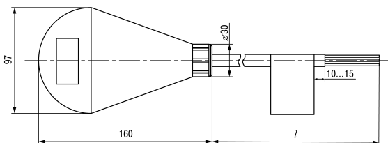
Рисунок 1.1 – Габаритные размеры
