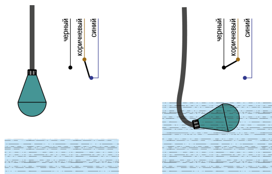
1) 2) Рисунок 4.1 – Переключение ПСУ
