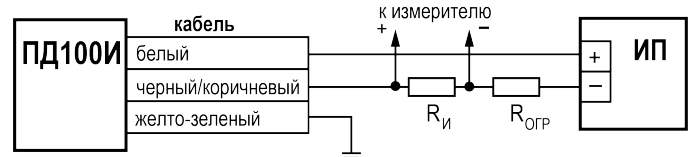
Рисунок 3 – Схема подключения
